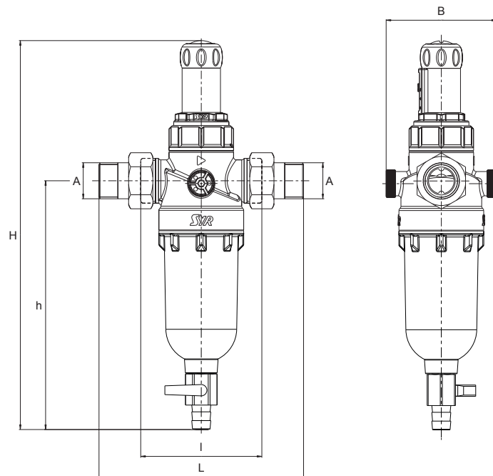
Ratio Start DFR filtr z ręcznym płukaniem wstecznym i reduktorem ciśnienia
